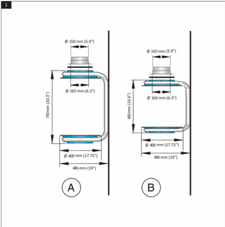
MFS dimensions
